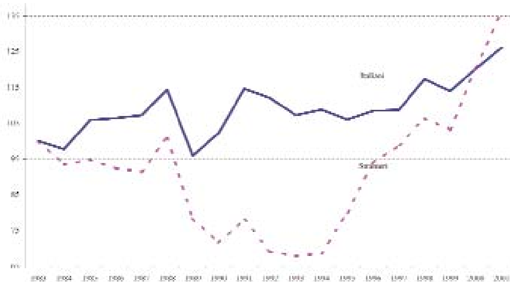
GRAF. 1.1.3 DINAMICA DELLE PRESENZE ITALIANE E STRANIERE IN ABRUZZO (1983=100)
